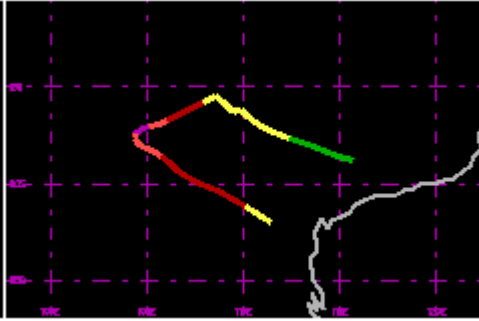
TC 19S Feb/Mar 1981 100kt
