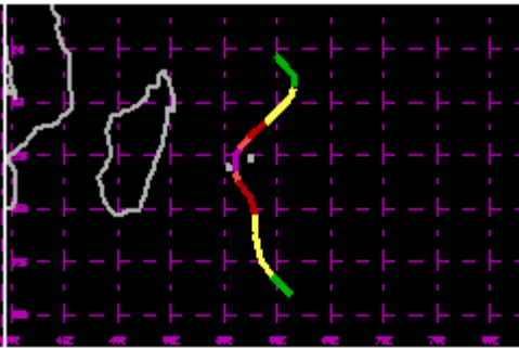
TC 08S Jan 1981 105kt
