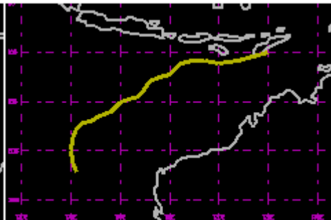
TC 06S Dec 1980 100kt
