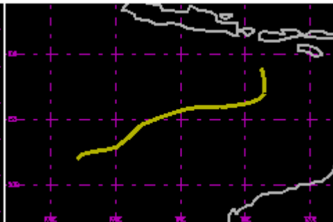
TC 04S Dec 1980 100kt
