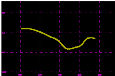
TC 01S Nov 1980 100kt
