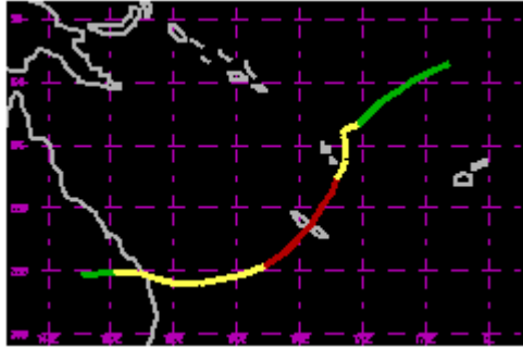
TC 15P Feb 1981 75kt
