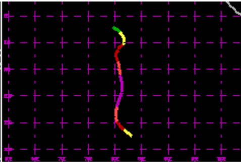
TC 05S Jan 1986 110kt
