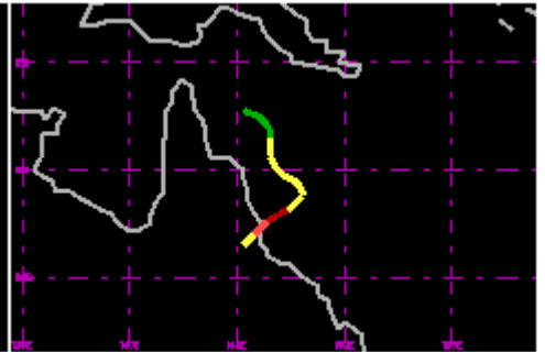
TC 12P Jan/Feb 1986 90kt
