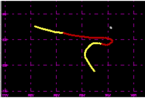
TC 15P Feb 1986 75kt
