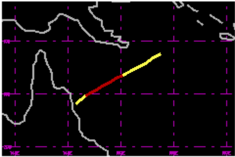
TC 31P Apr 1986 70kt
