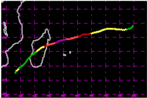
TC 25S Mar 1986 110kt
