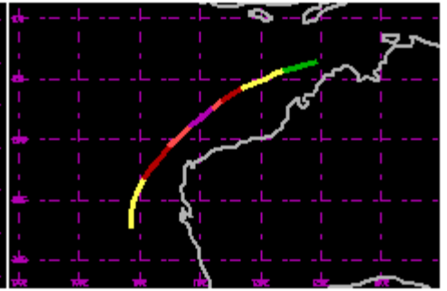
TC 22S Mar 1986 105kt
