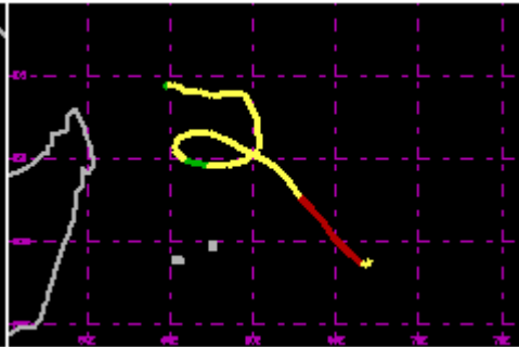
TC 06S Jan 1986 70kt
