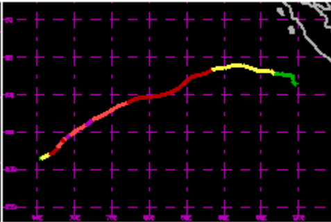
TC 02S Nov 1988 100kt
