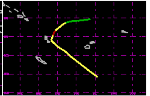
TC 30P Apr/May 1992 65kt
