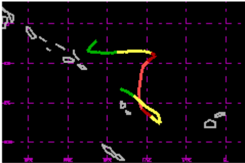
TC 03P Nov 1991 95kt
