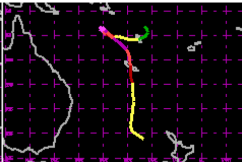
TC 24P Feb/Mar 1992 130kt
