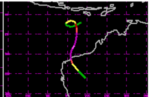
TC 23S Feb/Mar 1992 115kt
