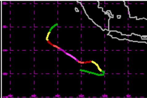
TC 05S Dec 1991 120kt
