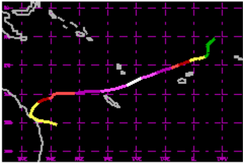
TC 25P Mar 1992 140kt
