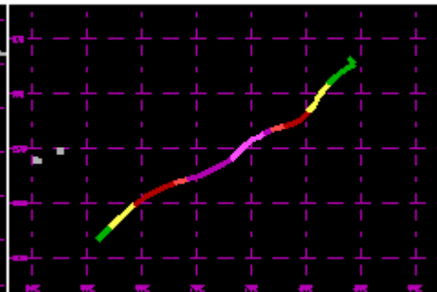
TC 22S Feb/Mar 1992 120kt
