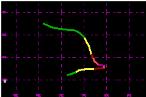
TC 09P Dec 1991 105kt
