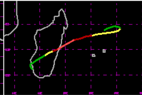
TC 08S Jan 1994 95kt
