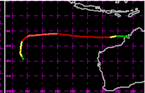
TC 09S Jan 1994 95kt
