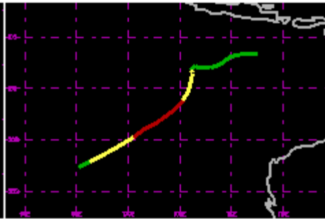
TC 12S Jan 1994 75kt
