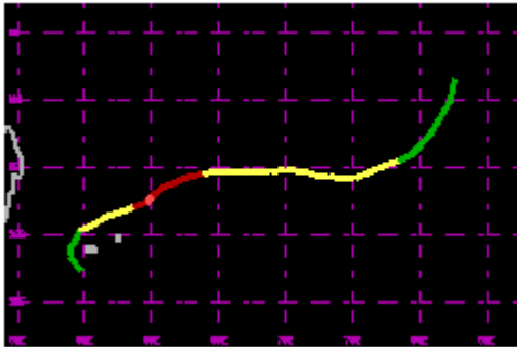
TC 03S Dec 1993 85kt
