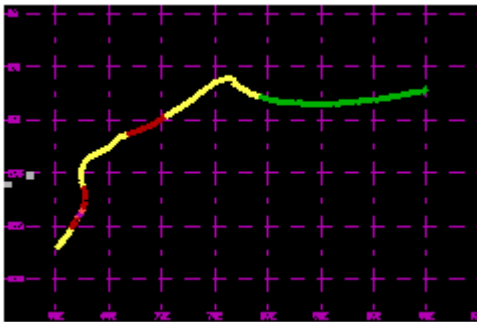
TC 16S Feb 1994 100kt
