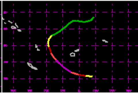
TC 24P Mar 1994 105kt
