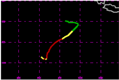
TC 04S Nov 1998 70kt
