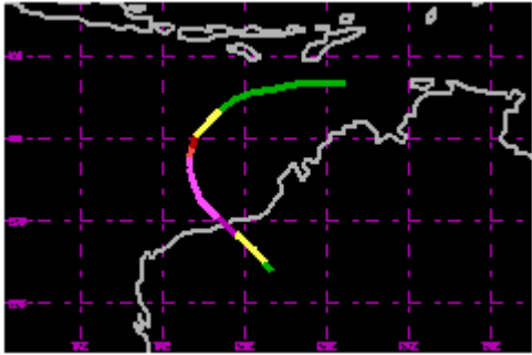
TC 32S Apr 1999 130kt
