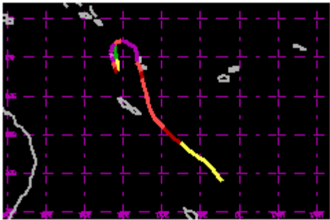
TC 11P Jan 1999 115kt
