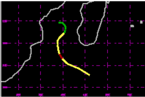
TC 12S Jan 1999 65kt
