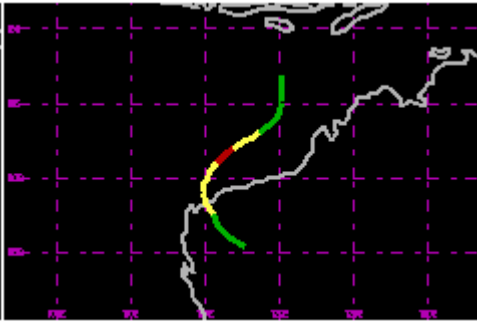
TC 05S Dec 1998 65kt
