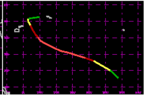
TC 09P Dec 1998 90kt
