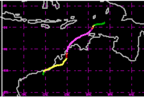
TC 06S Dec 1998 135kt
