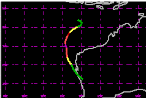
TC 28S Mar 1999 100kt
