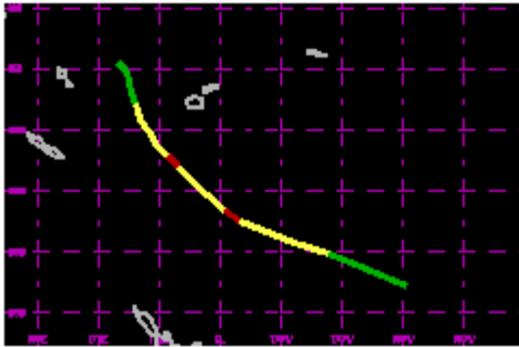
TC 07P Jan 2000 65kt
