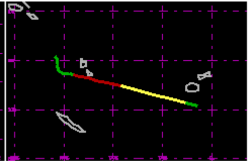
TC 05P Jan 2000 70kt
