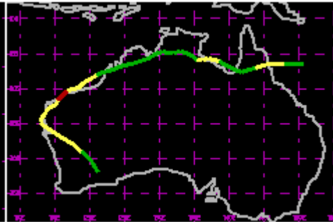
TC 14P Feb/Mar 2000 65kt
