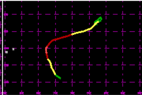
TC 04S Jan 2000 90kt
