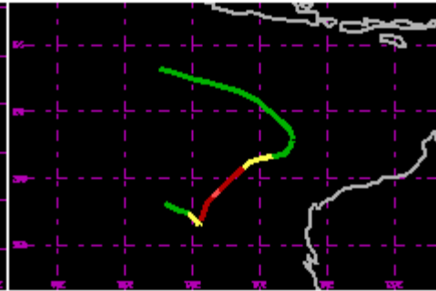
TC 09S Jan 2000 85kt
