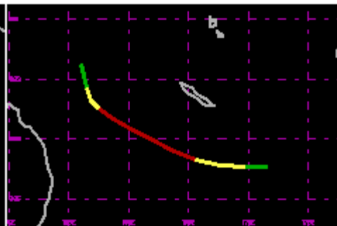
TC 14P Feb 2002 75kt
