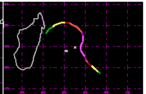
TC 15S Mar 2002 120kt
