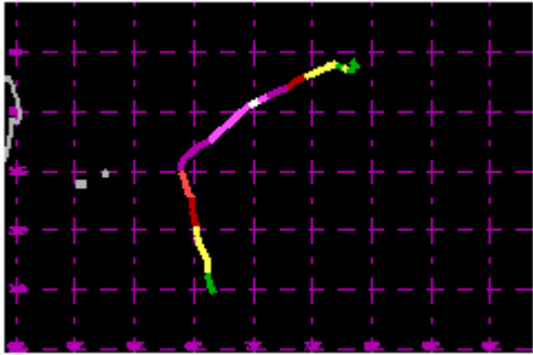
TC 23S Mar 2003 140kt
