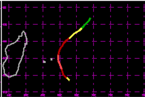
TC 05S Dec 2002 90kt
