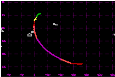
TC 10P Jan 2003 110kt
