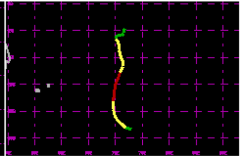
TC 09S Jan 2003 65kt
