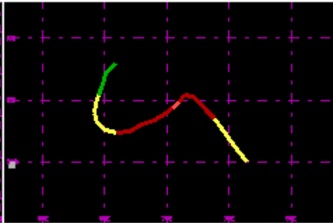
TC 17S Feb 2003 90kt
