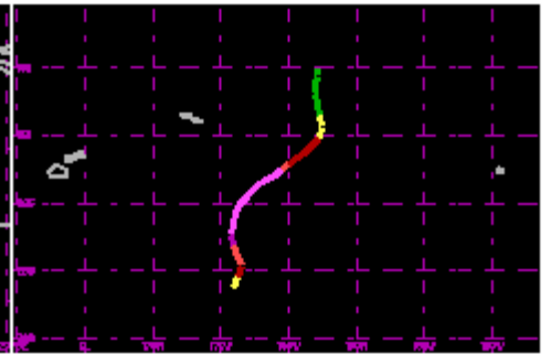
TC 15P Feb 2003 130kt
