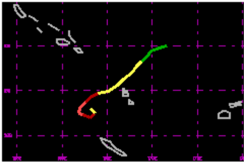
TC 29P Jun 2003 90kt
