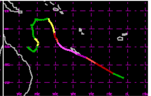
TC 22P Mar 2003 130kt
