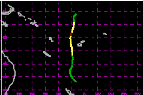
TC 03P Nov 1977 65kt
