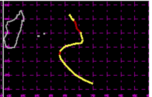
TC 09S Jan 1987 75kt
