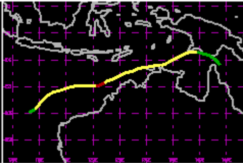
TC 23P Apr 1987 65kt
