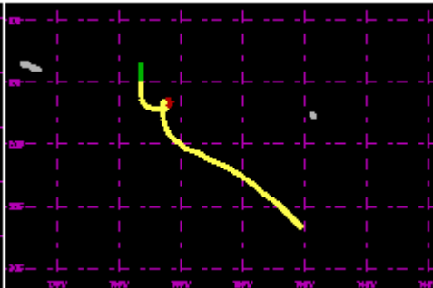
TC 05P Dec/Jan 1987 65kt
