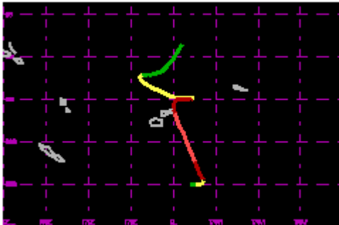
TC 04P Dec 1986 90kt
