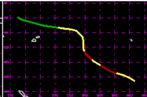
TC 20P Feb/Mar 1987 65kt
