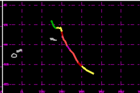
TC 08P Jan 1987 100kt
