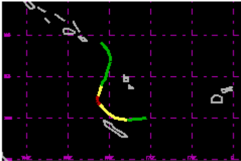
TC 22P Mar 1987 65kt
