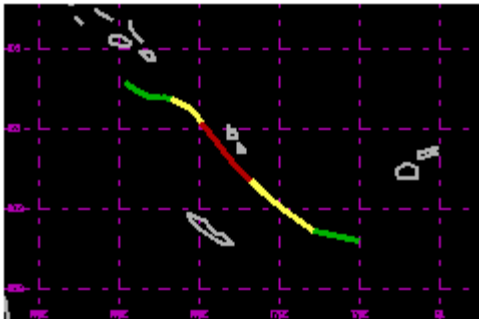
TC 14P Feb 1987 75kt
