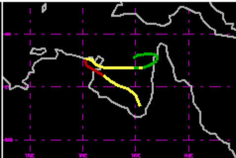
TC 15P Feb 1987 65kt
