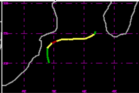
TC 21S Jun 2001 65kt
