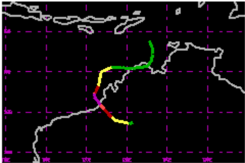
TC 03S Dec 2000 110kt
