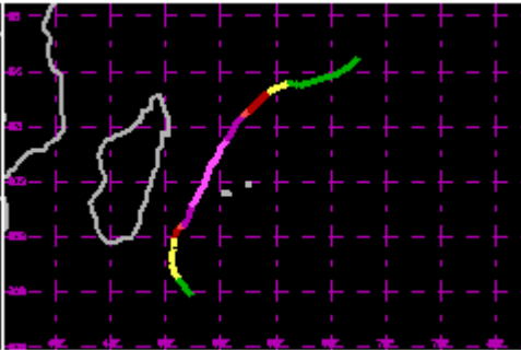
TC 04S Jan 2001 120kt
