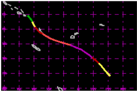
TC 13P Feb/Mar 2001 105kt
