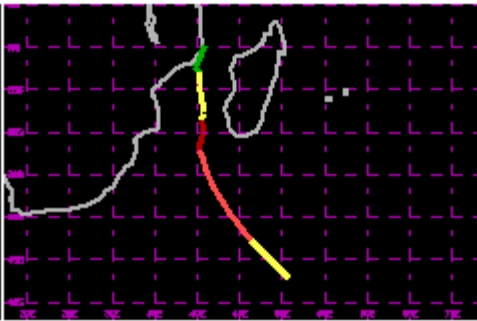
TC 15S Mar 2000 90kt
